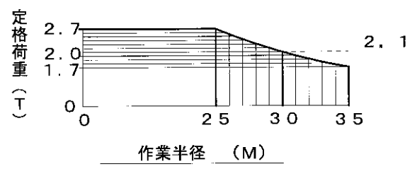
定格荷重曲線表
