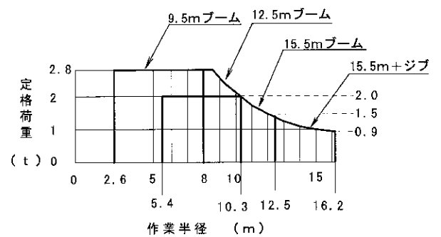
性能曲線図
