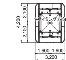
B矢視 (外部建設時)
