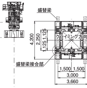
盛替梁接合部平面図
