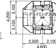
A矢視
