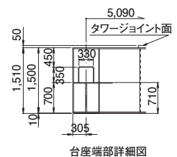
台座端部詳細図
