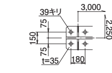
盛替梁接合部詳細図
