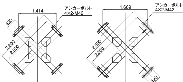
平台座 3段自立型
