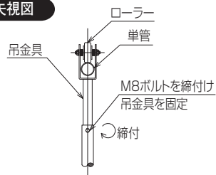
B矢視図
