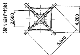
□台座平面図 (単位: mm)
