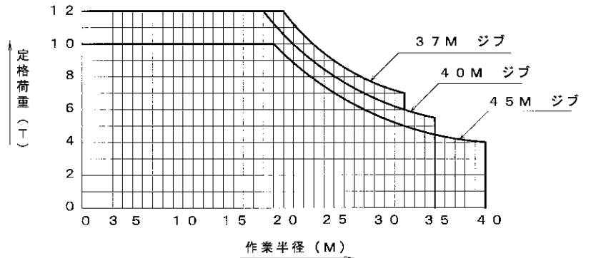
性能線図
