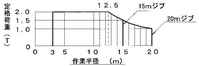
性能曲線図
