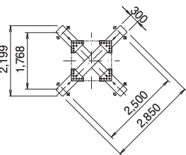
台座平面図 7段自立型
