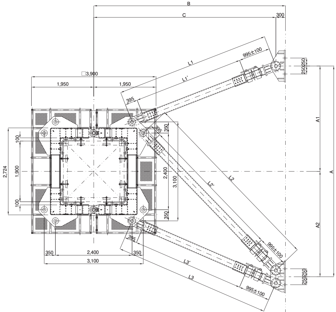
□主要寸法図 (単位: mm)
