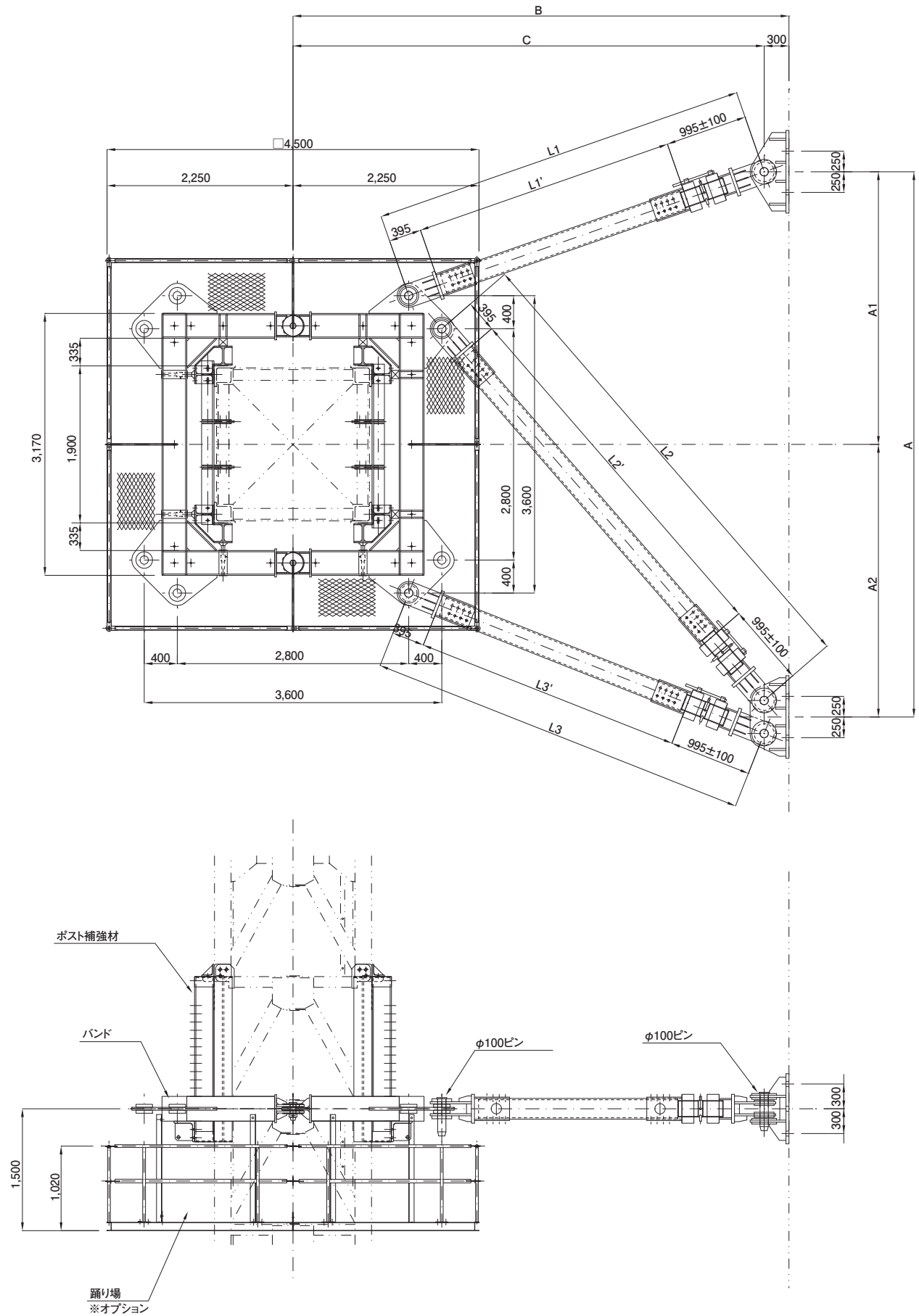
□主要寸法図 (単位: mm)
