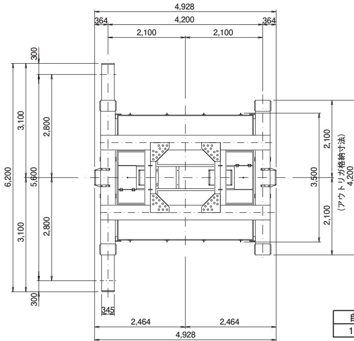
□主要寸法図 (単位: mm)
