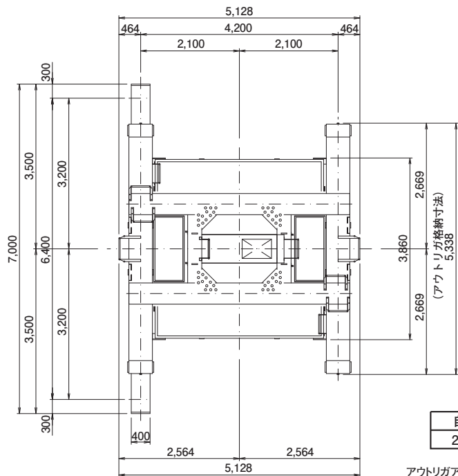
□主要寸法図 (単位: mm)
